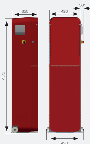
Terminal con armario
