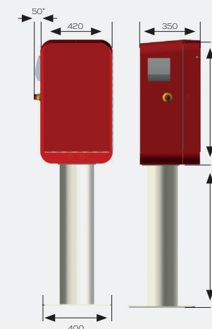
Terminal con pedestal
